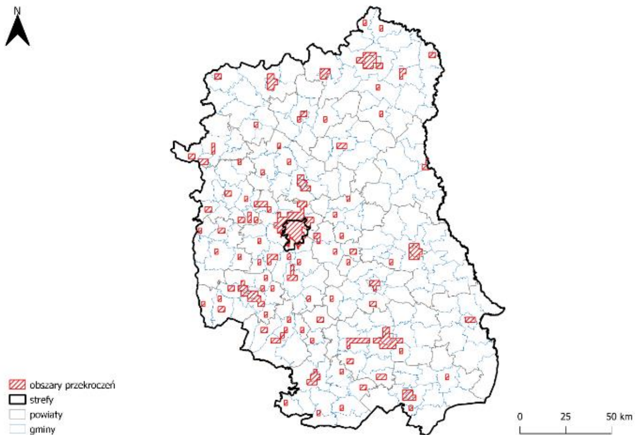
Mapa 4 Zasięg obszarów przekroczeń poziomu docelowego stężenia B(a)P określonego ze względu na ochronę zdrowia ludzi w województwie lubelskim w 2021 r.
